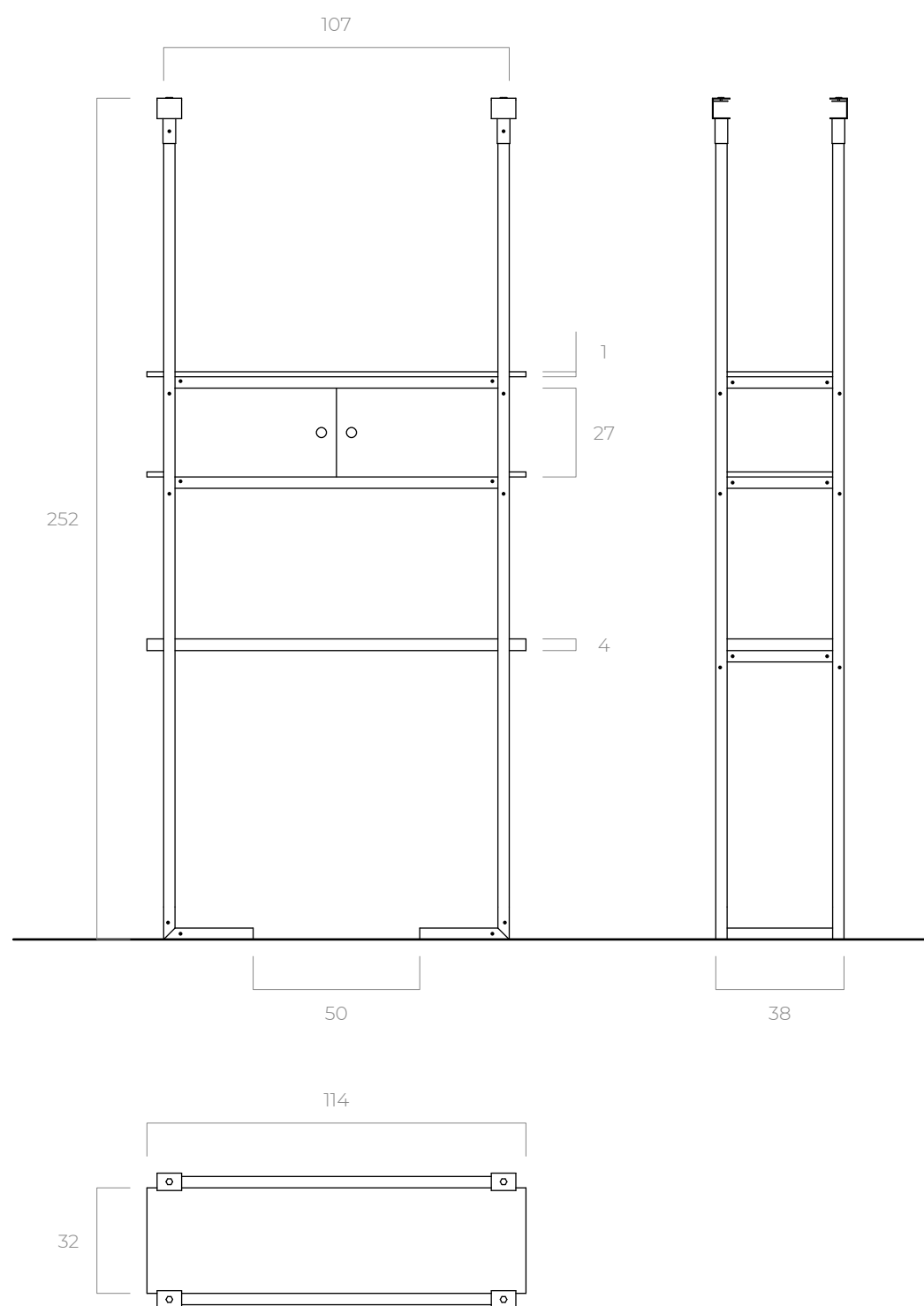
Mobile fermata Relax showroom scala 1:20 unità di misura: cm
