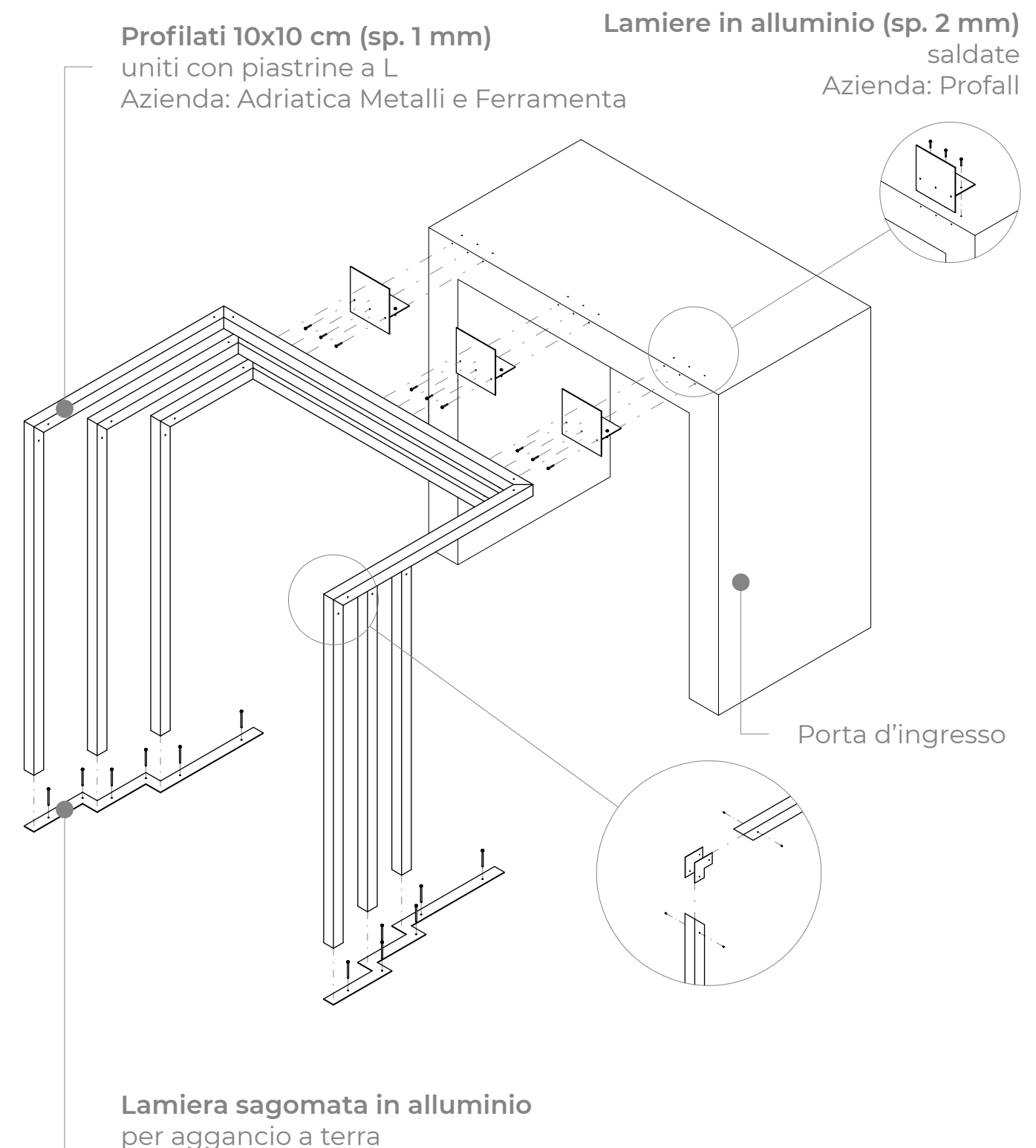
Esploso assonometrico scala 1:50
